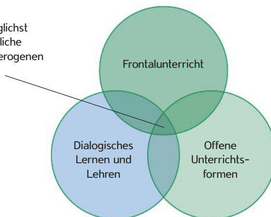
Venn-Diagramm
